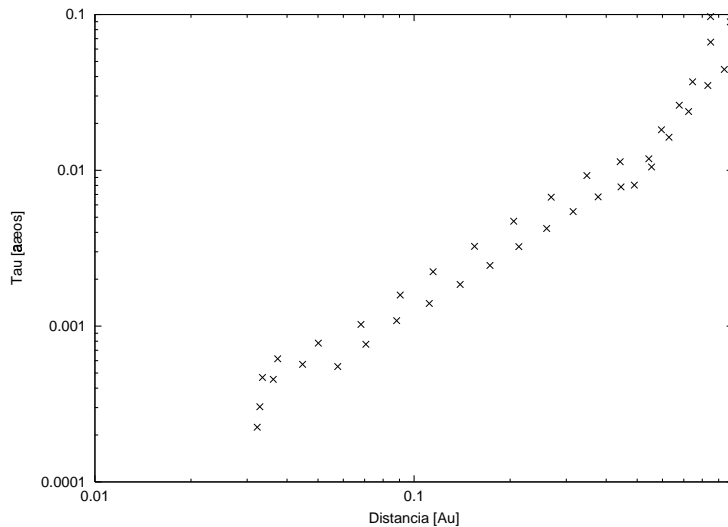
Figura 8.8: Paso de tiempo como función de la distancia radial desde el programa orbita usando el método de Runge-Kutta adaptativo. Los parámetros son los mismos de la figura 8.7.
