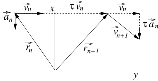
Figura 6.1: Trayectoria de una partícula después de un único paso de tiempo con el método de Euler. Sólo para efectos ilustrativos \tau es grande.
