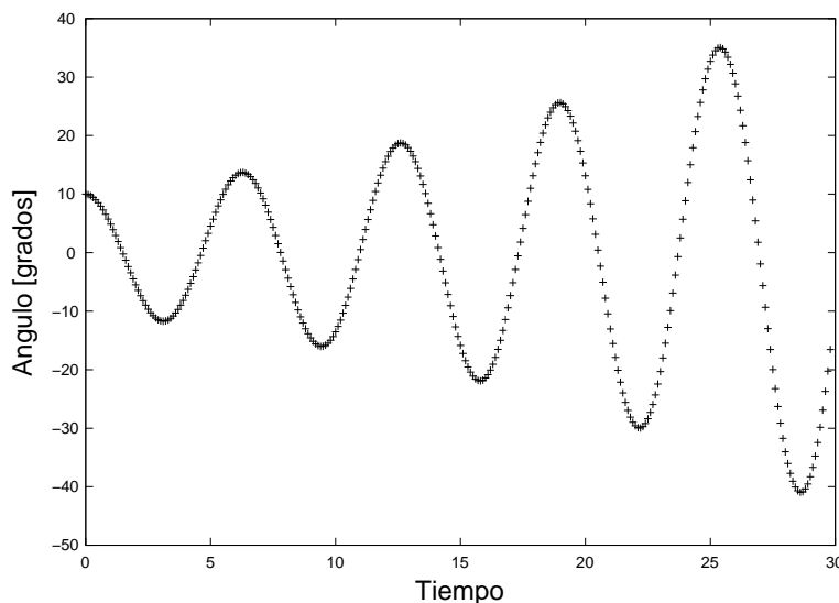
Figura 6.4: Salida del programa péndulo usando el método de Euler. El ángulo inicial es \theta_m = 10^\circ , el paso en el tiempo es \tau = 0.1 , y 300 iteraciones fueron calculadas.
